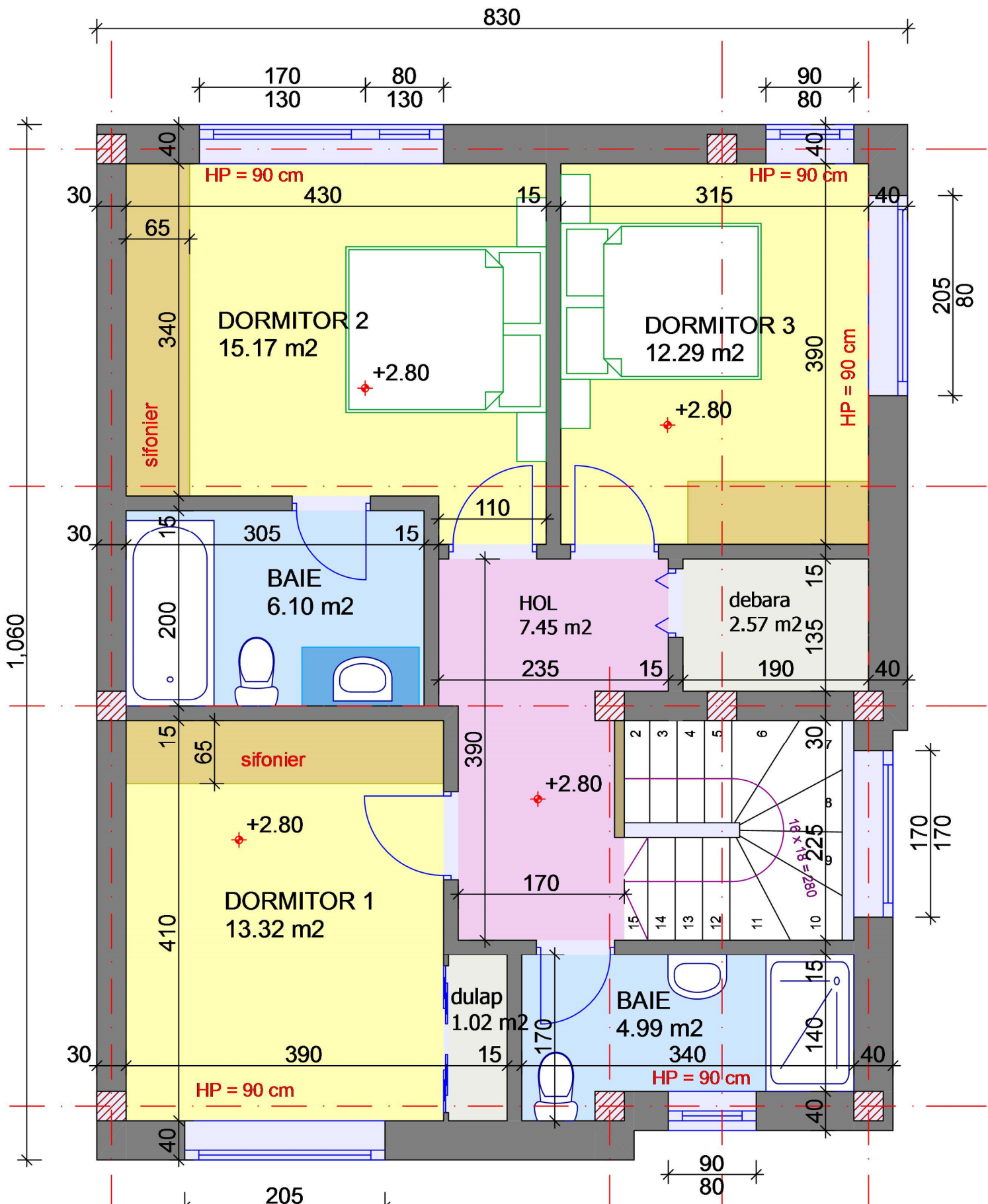
PLAN ETAJ A: 86.53 m 2
