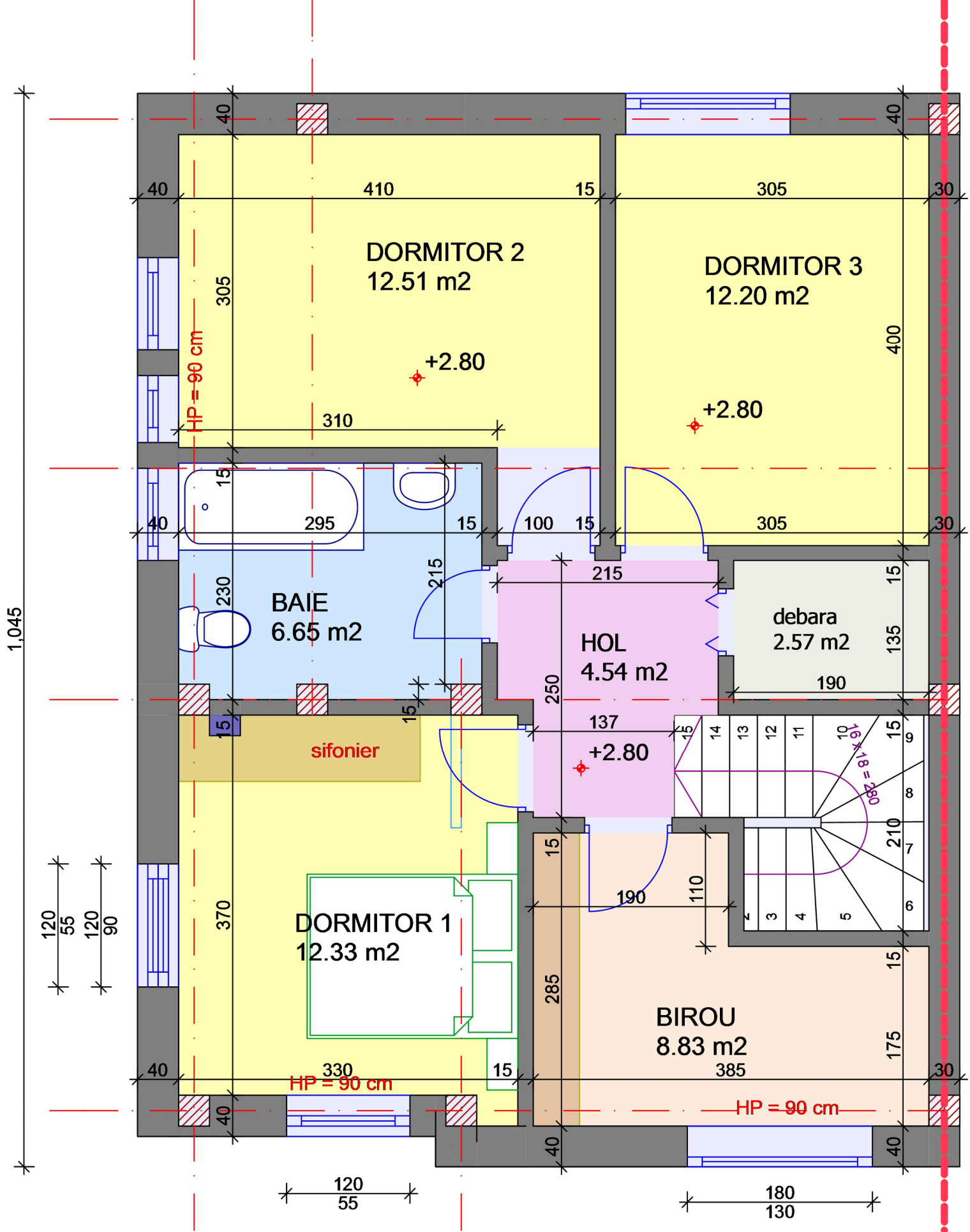
PLAN ETAJ A: 81.16 m 2
